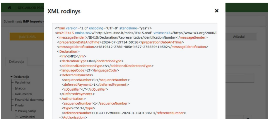
pav. 29 Deklaracijos XML rodinys
