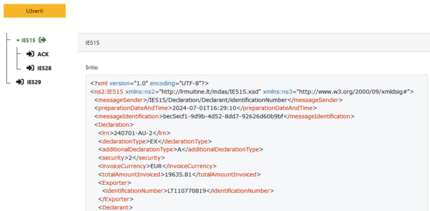
pav. 87 Su deklaracija susijusių pranešimų peržiūros langas
